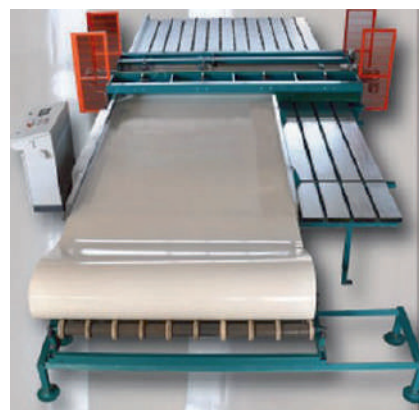
Tagliatrice di laminati a dimensioni programmate completamente automatica di totale creazione VMC Srl.
